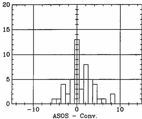
ASOS - Conv. (DeltaT)- ALS 8 1993
