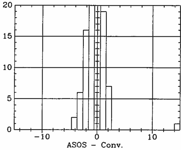
ASOS - Conv. (DeltaT)- AMA 8 1993
