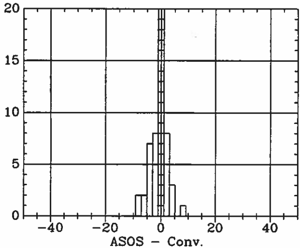
ASOS - Conv. (RH)- ALS 7 1993
