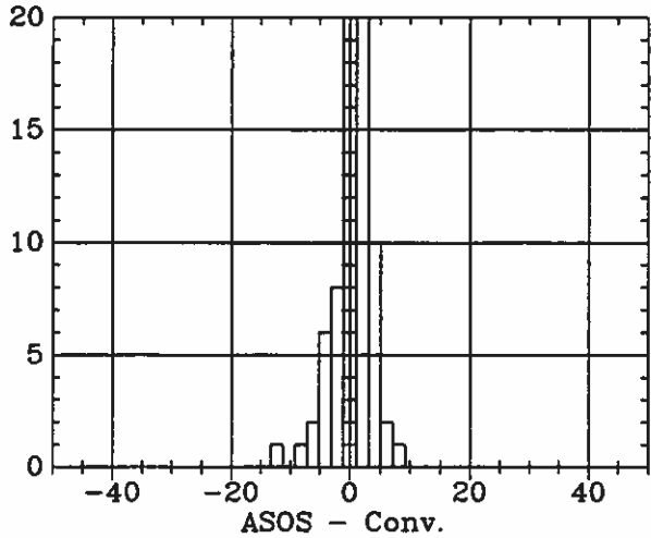
ASOS - Conv. (RH)- AMA 7 1993
