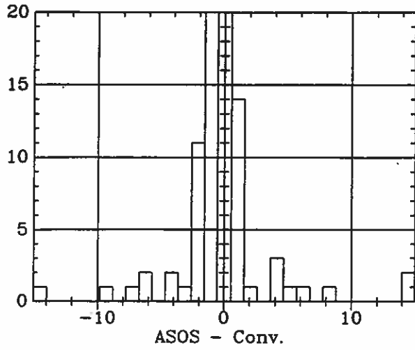
ASOS - Conv. (DeltaT)- AMA 8 1993
