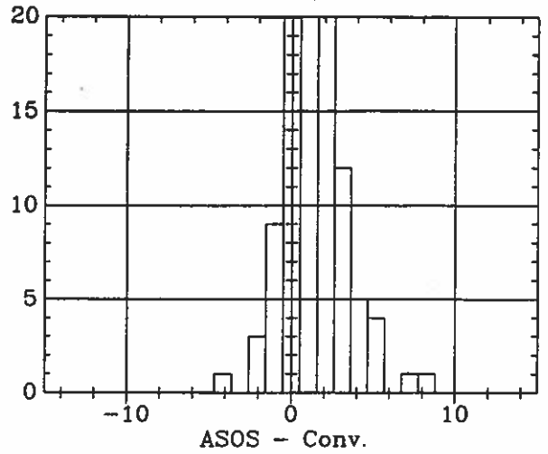
ASOS - Conv. (RH)- TOP 6 1993
