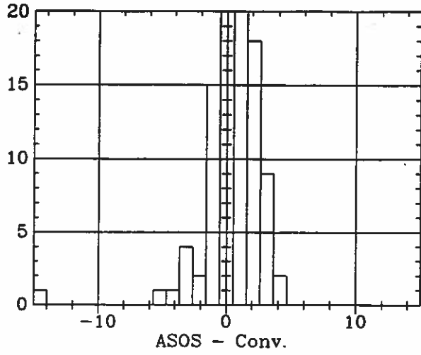
ASOS - Conv. (DeltaT)- TOP 8 1993
