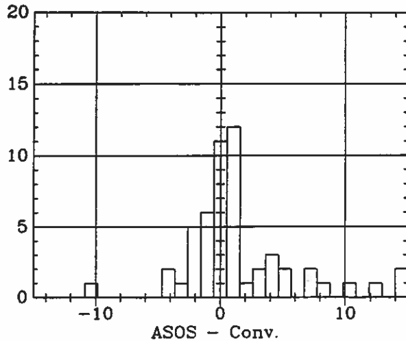
ASOS - Conv. (RH)- ALS 6 1993
