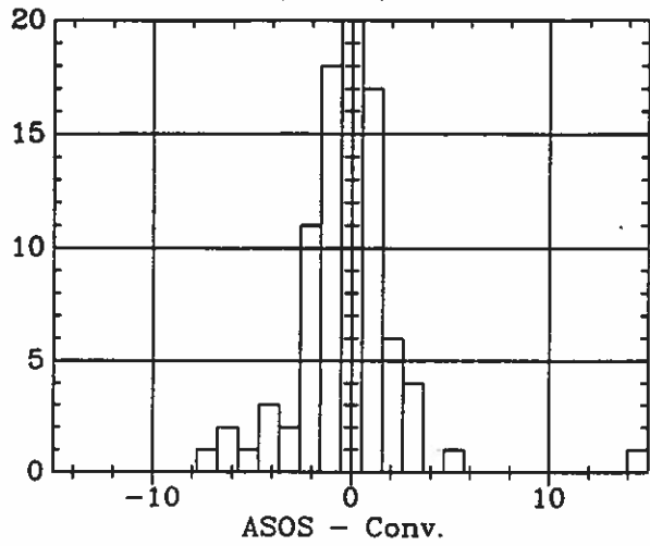
ASOS - Conv. (DeltaT)- GRI 8 1993
