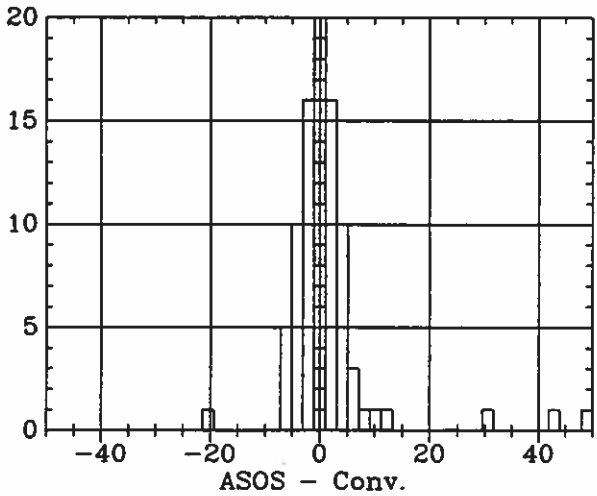
ASOS - Conv. (RH)- GRI 7 1993
