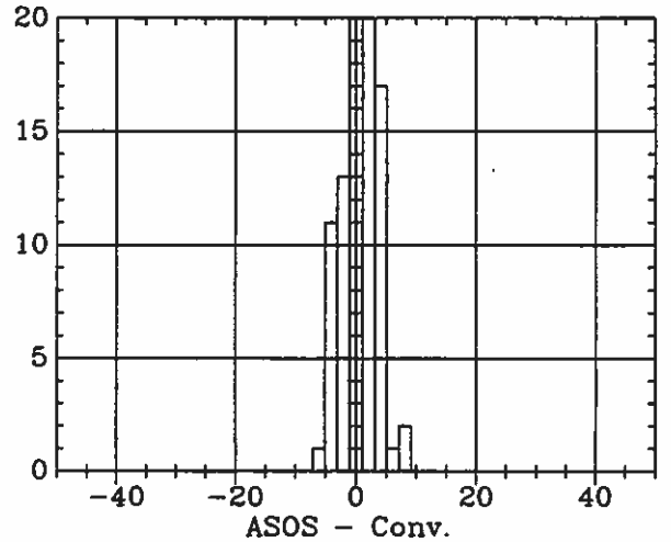
ASOS - Conv. (RH)- AMA 8 1993
