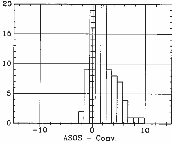
ASOS - Conv. (DeltaT)- TOP 8 1993
