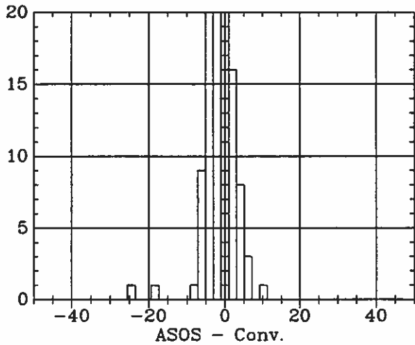
ASOS - Conv. (RH)- DDC 7 1993
